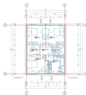
RZUT PODDASZA
