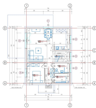
RZUT PARTERU
